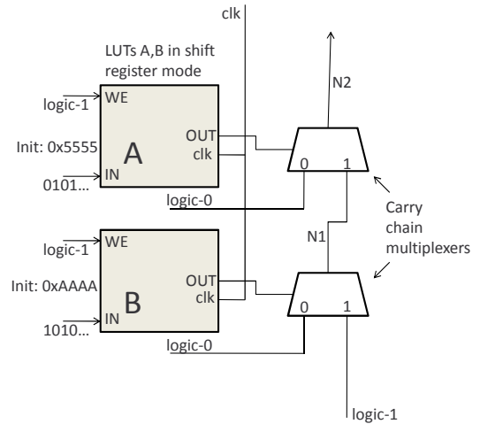
Fig. 3. PUF circuit.
